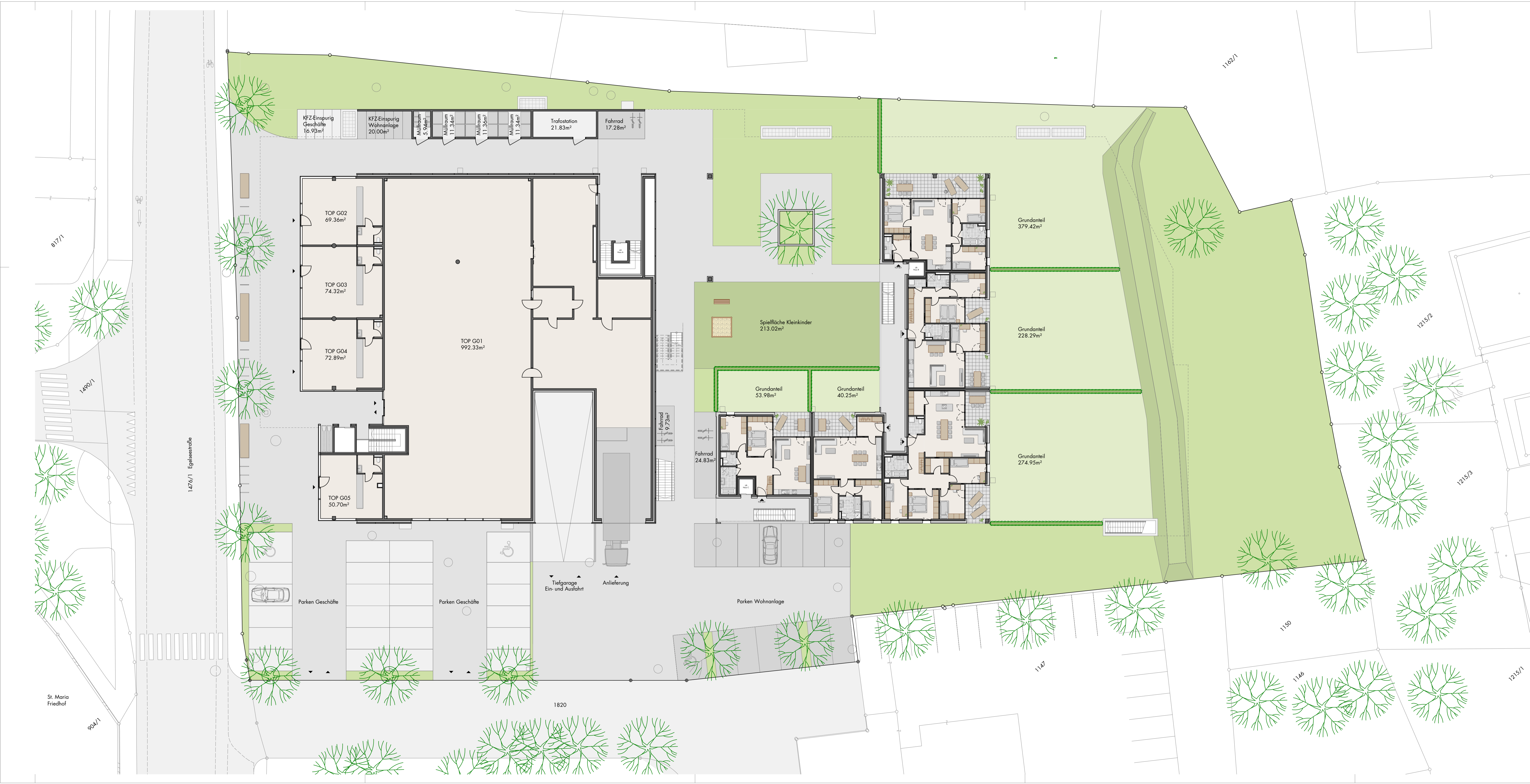
Übersichtsplan 1:200
