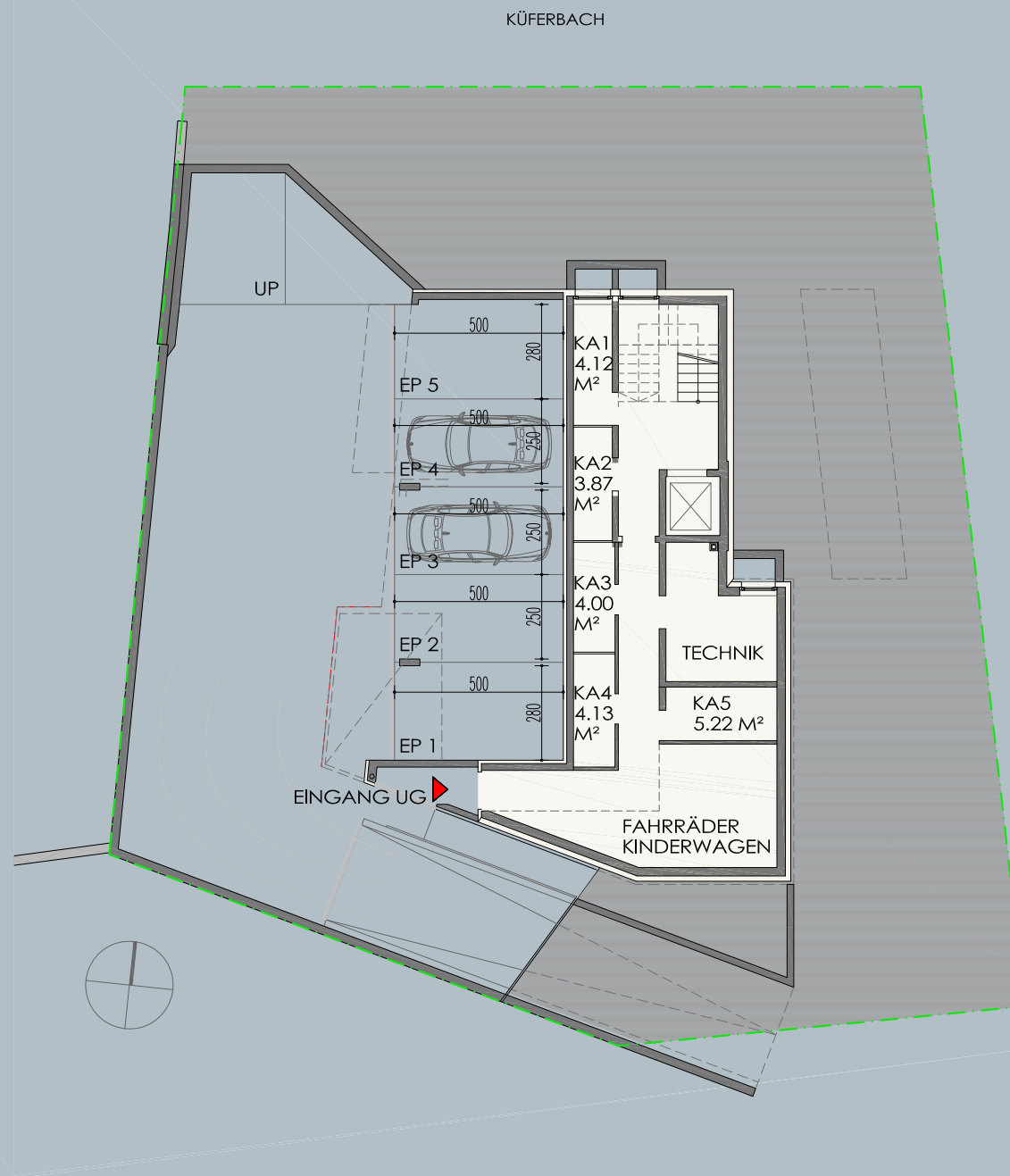
UNTERGESCHOSS 1:200
