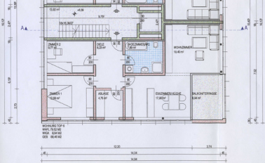
GRUNDRISS OBERGESCHOSS 2 1:100
