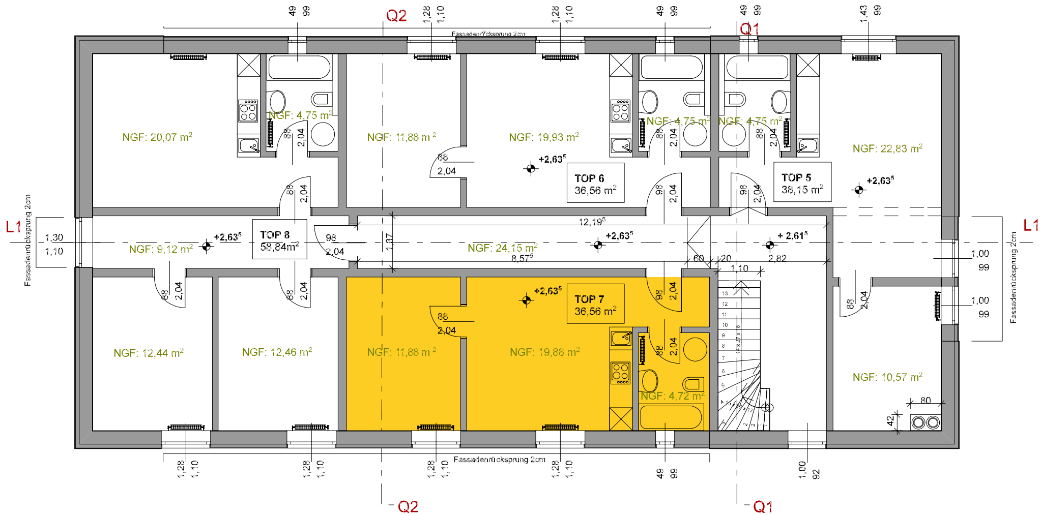
OBERGESCHOSS 1/100
