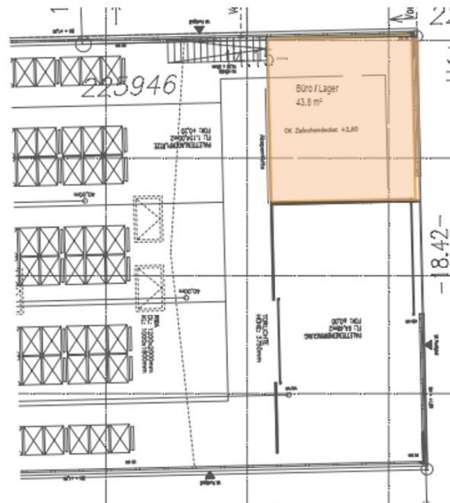
Grundriss Obergeschoss
