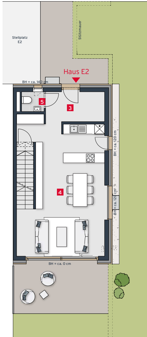
ERDGESCHOSS
