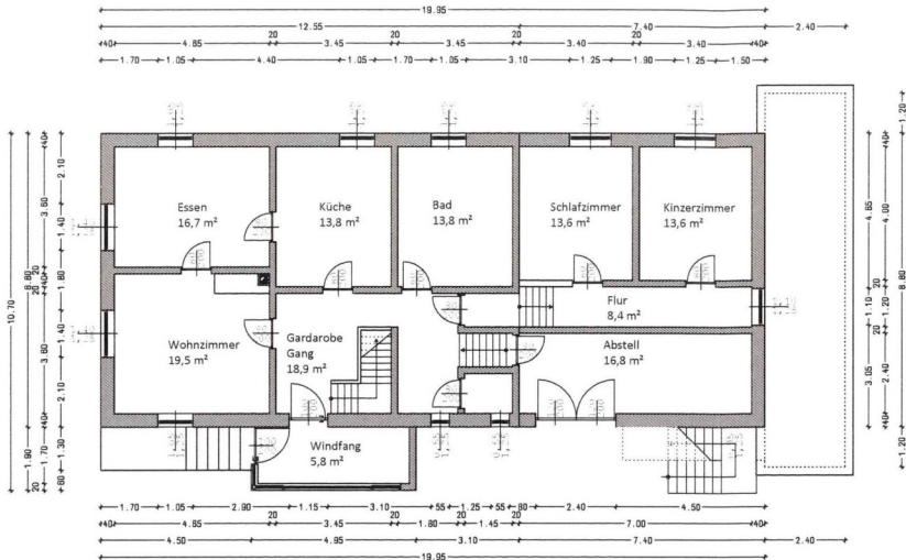
Erdgeschoss 1:100
