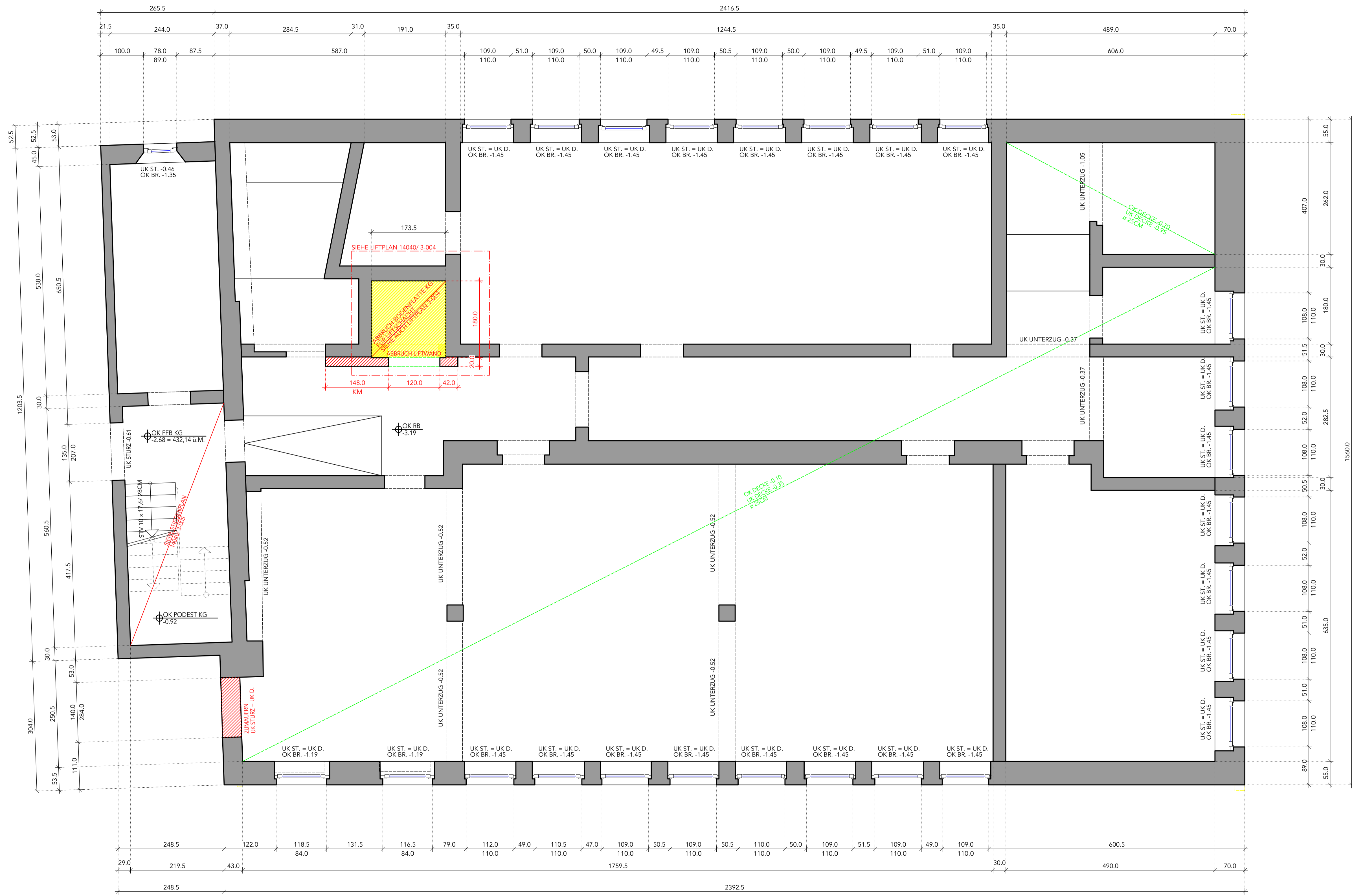
GRUNDRISS KELLERGESCHOSS M 1:50
