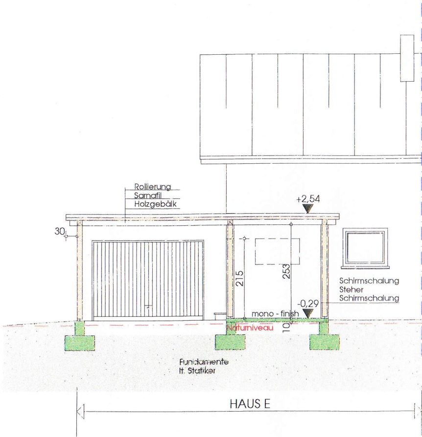
Höhenschnitt B- B
