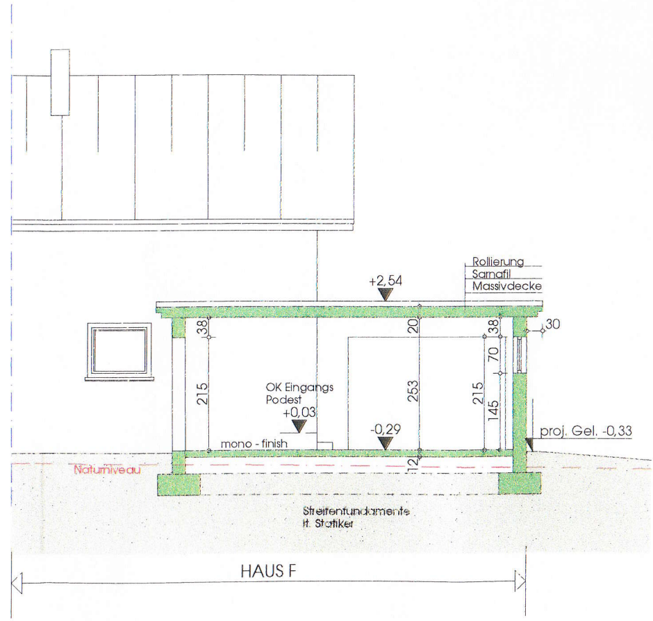
Höhenschnitt C- C
