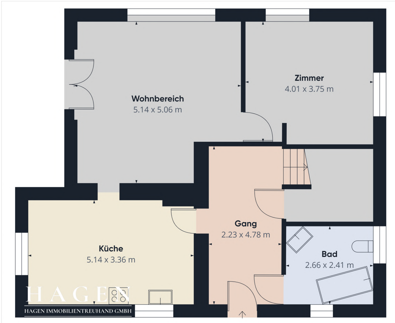
Grundrissplan ohne Maßstab EG
