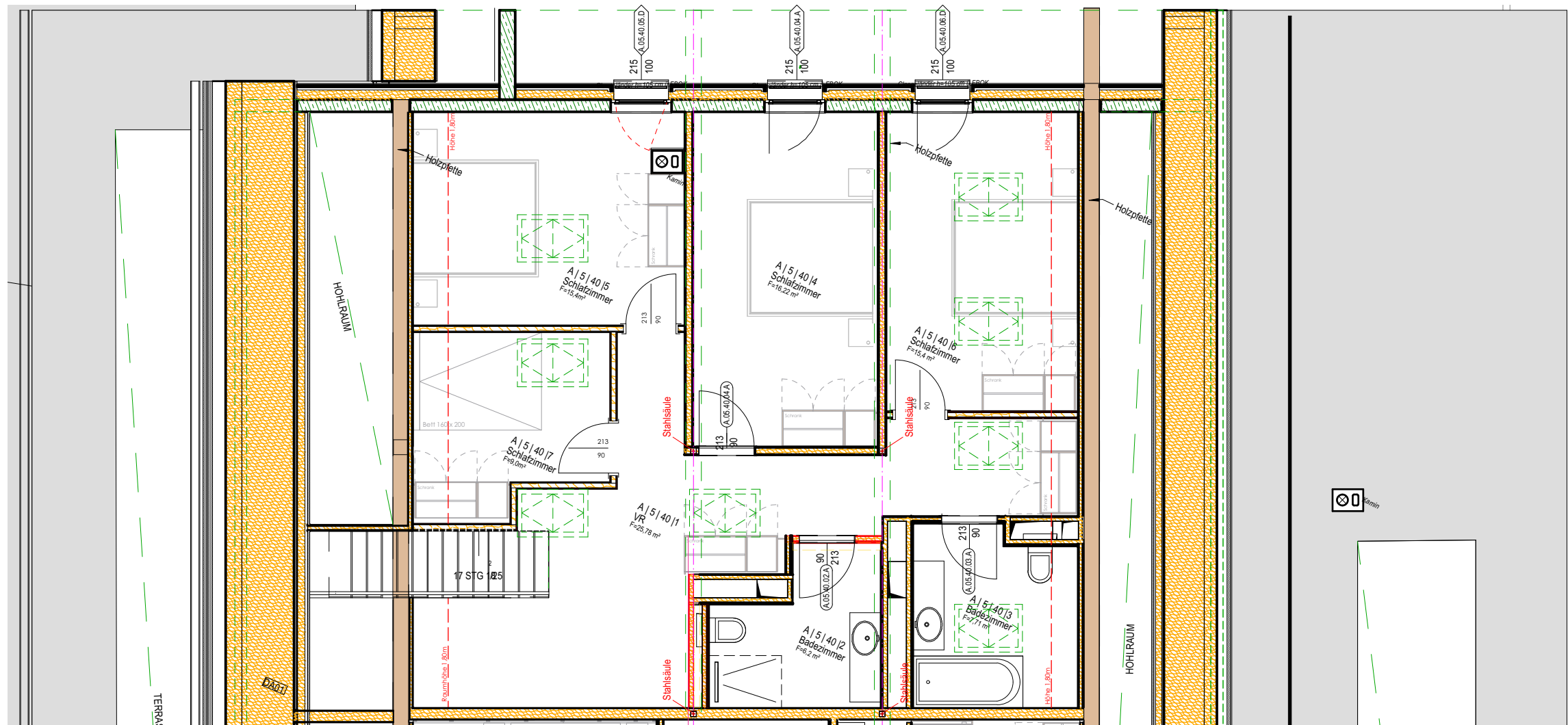
Grundriss 5. Obergeschoss
