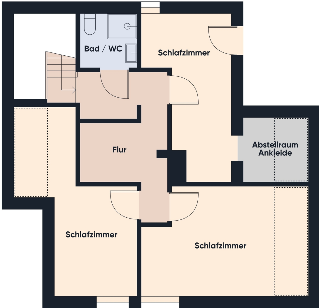
Grundriss DG
