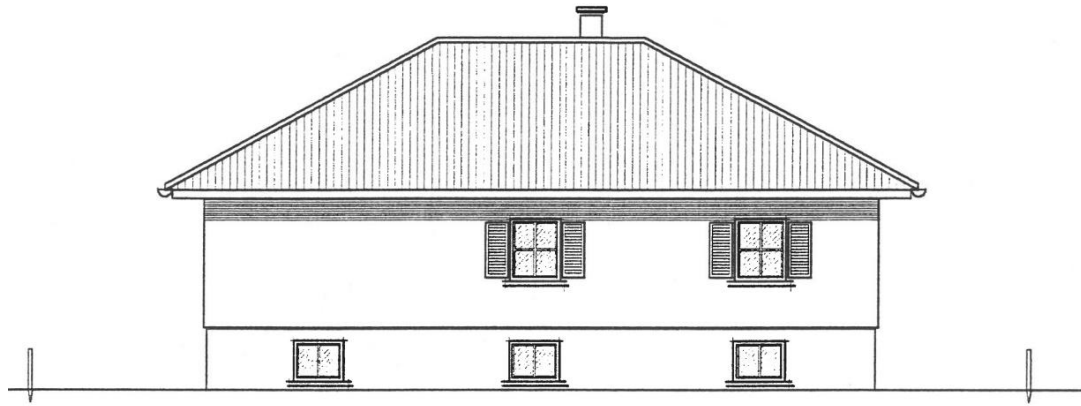
Ostansicht
