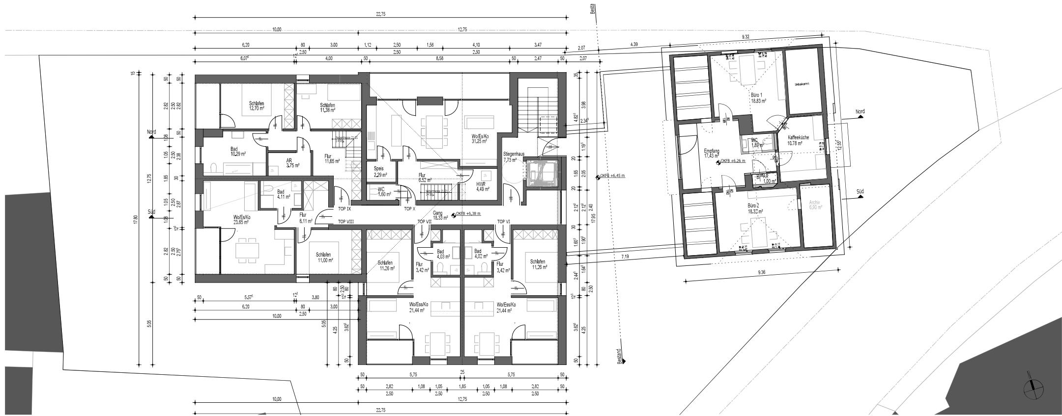
2. OBERGESCHOSS
