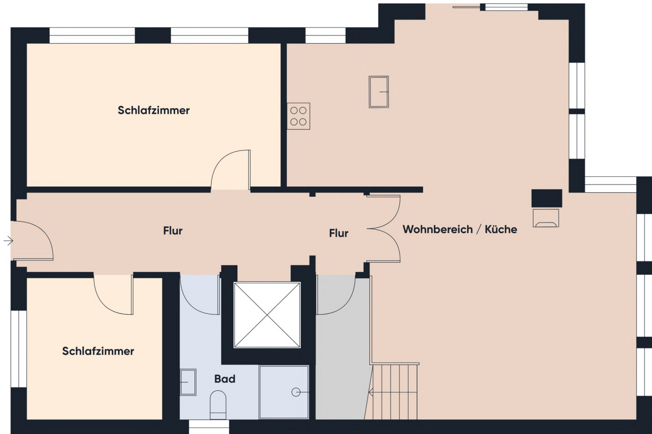
Grundrissplan ohne Maßstab EG
