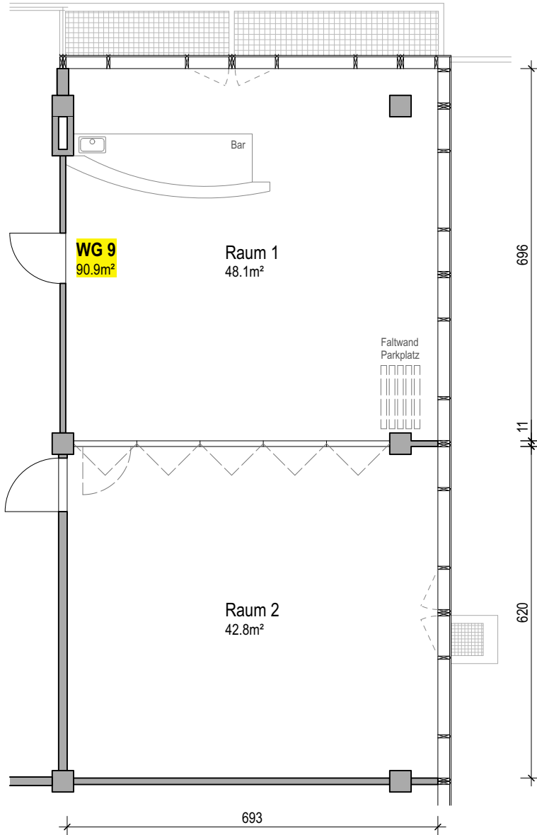
Grundriss
