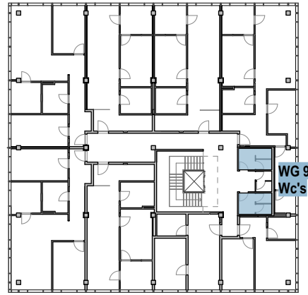
Übersichtsplan 1. OG
