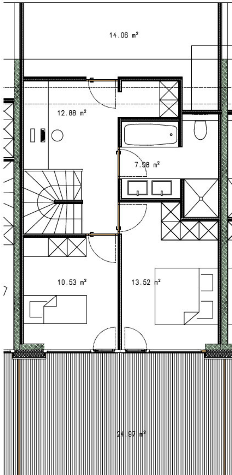
Grundrissplan Dachgeschoß
