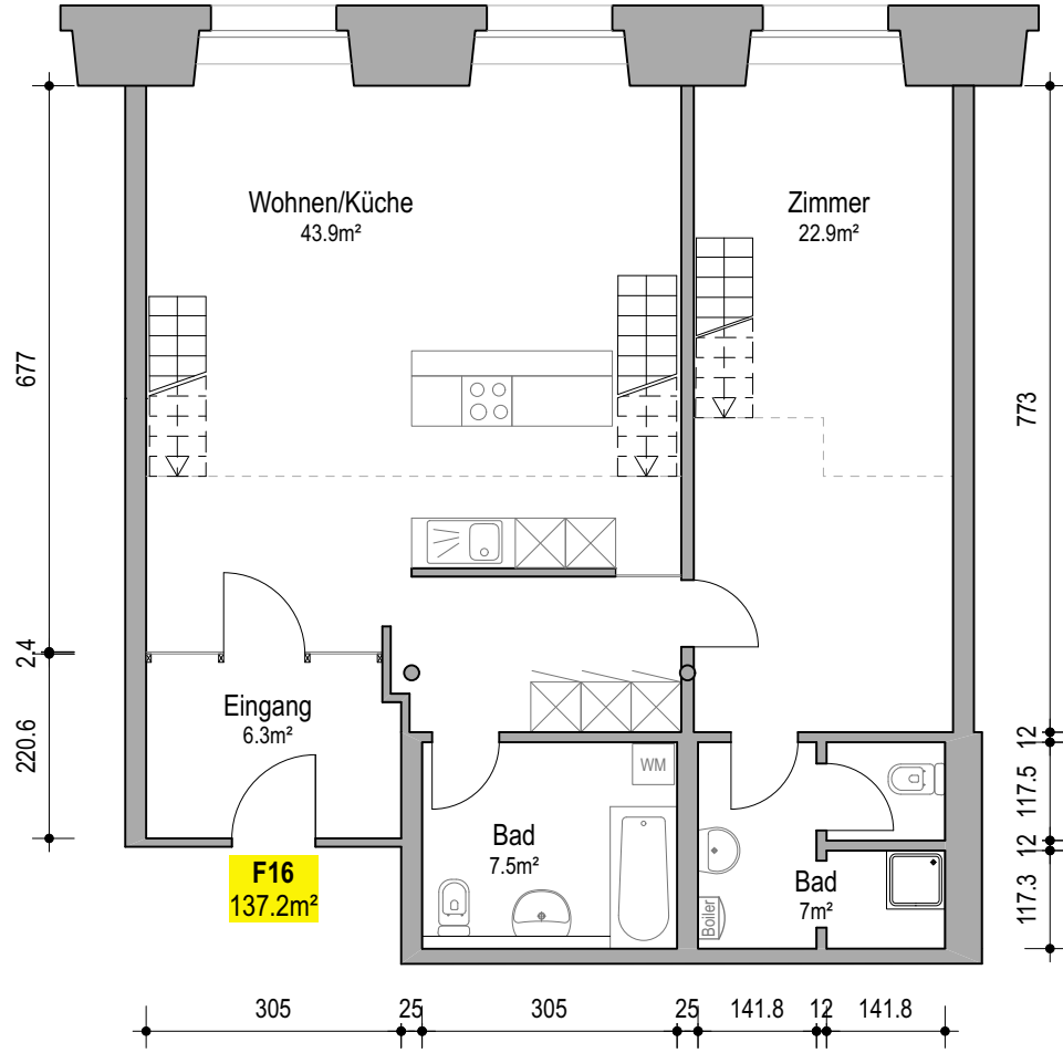
Top F16 Wohnung Mst. 1:100
