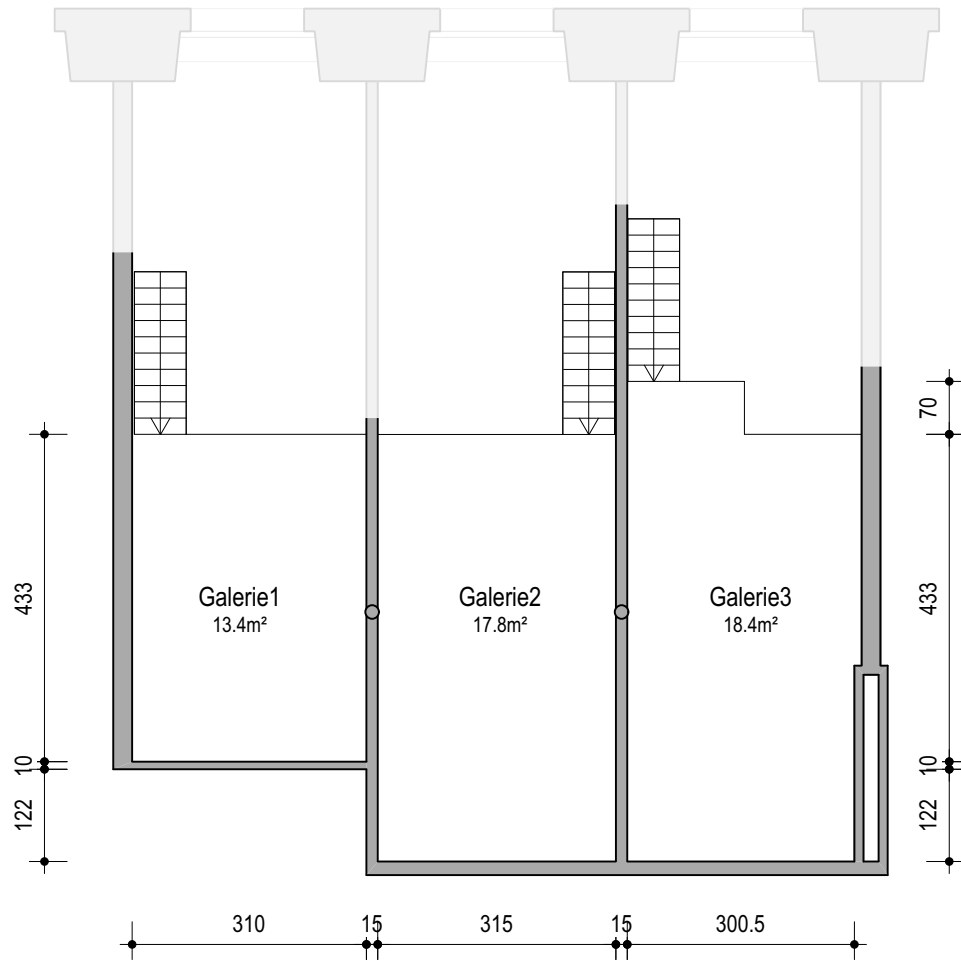
Top F16 Galerie Mst. 1:100
