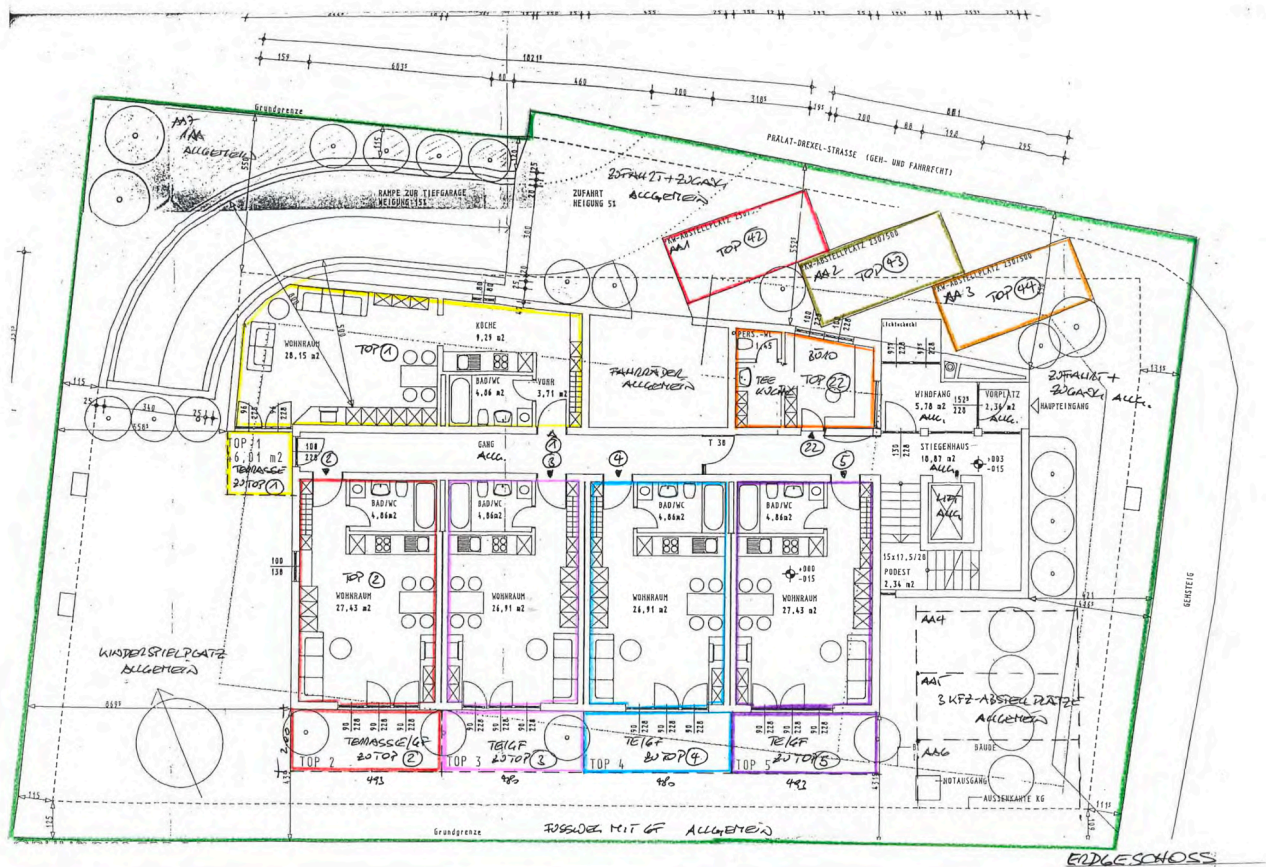
Grundrissplan ohne Maßstab EG
