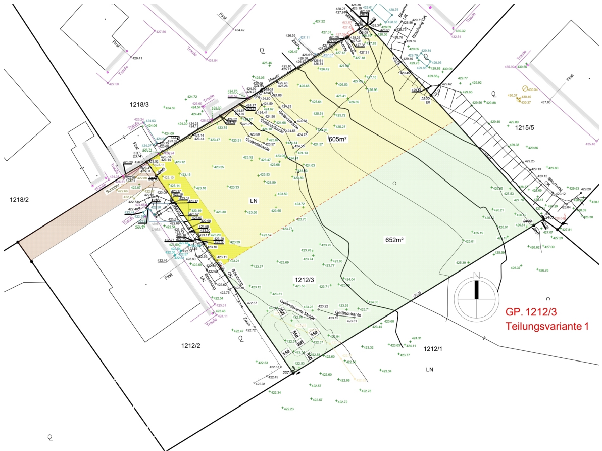
Teilungsvariante 1
