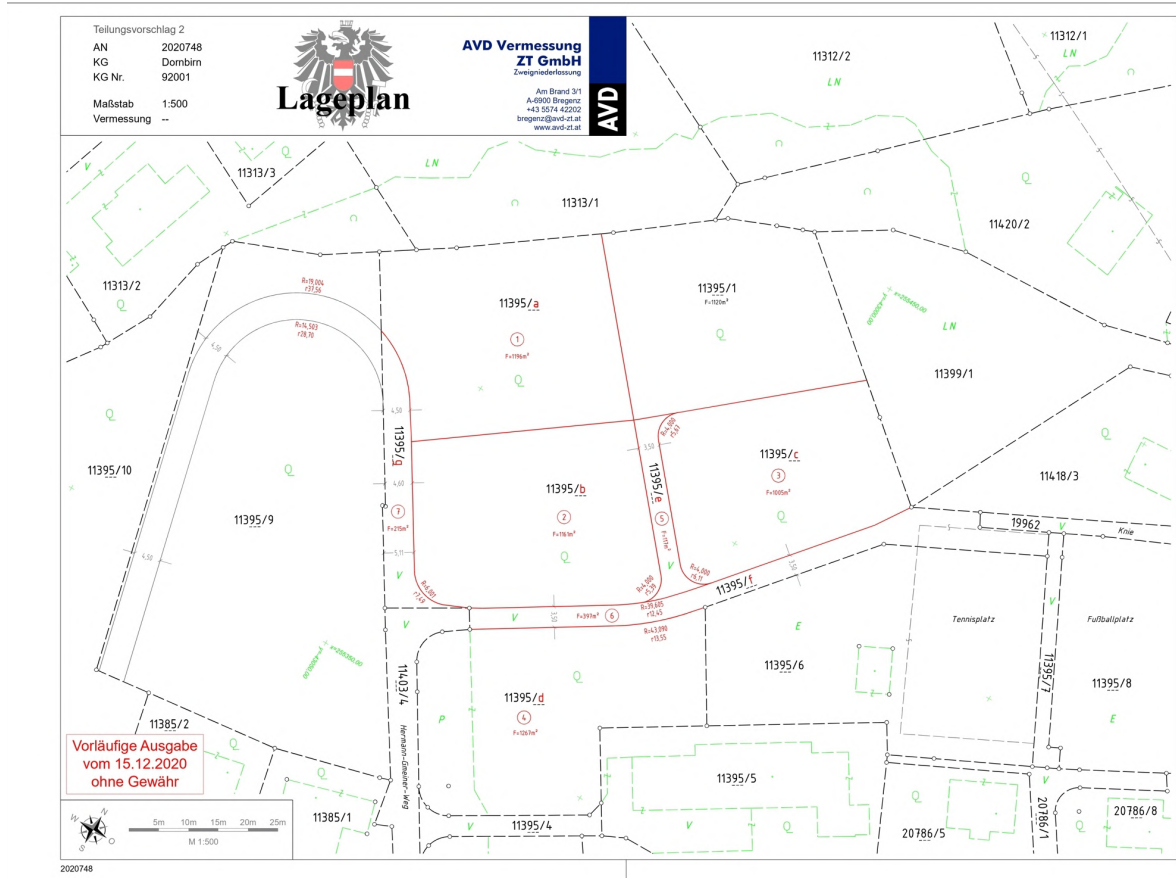
Teilungsvorschlag
