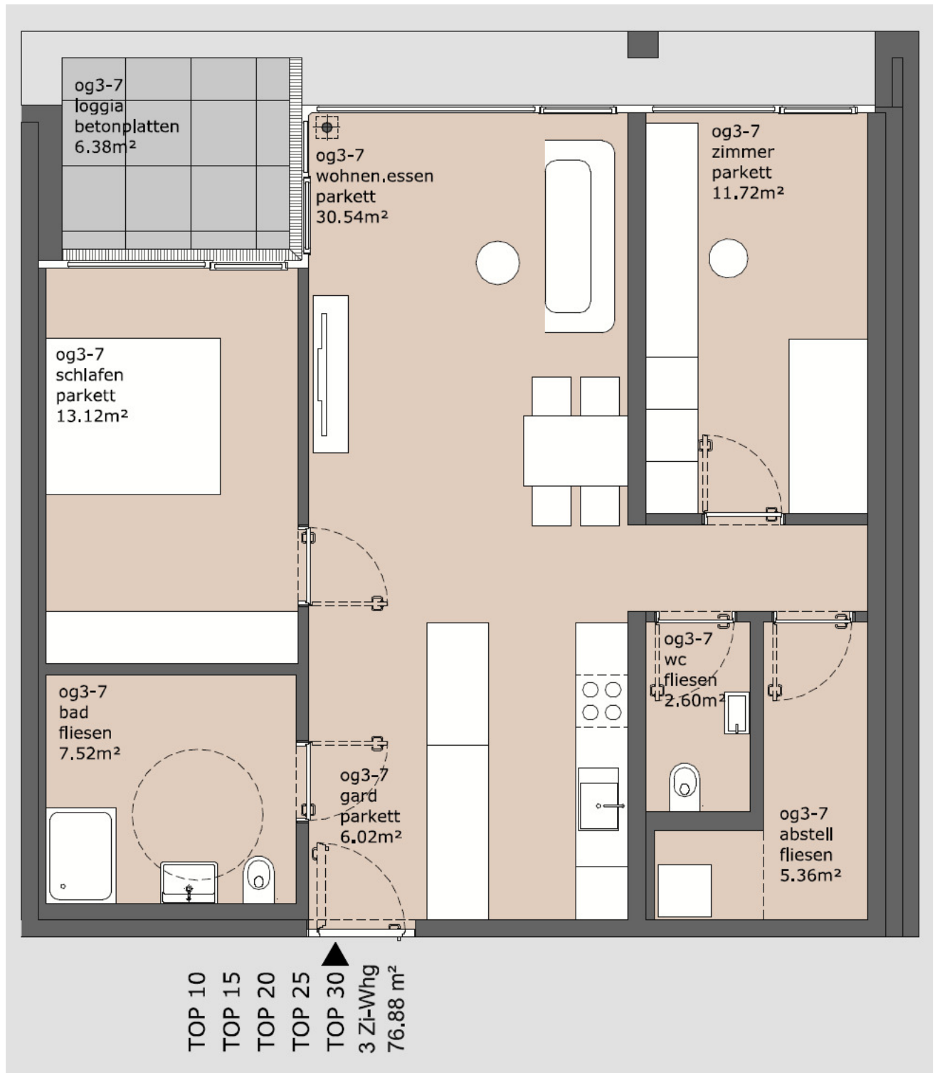
Grundriss der Tops 10, 15, 20, 25 und 30
