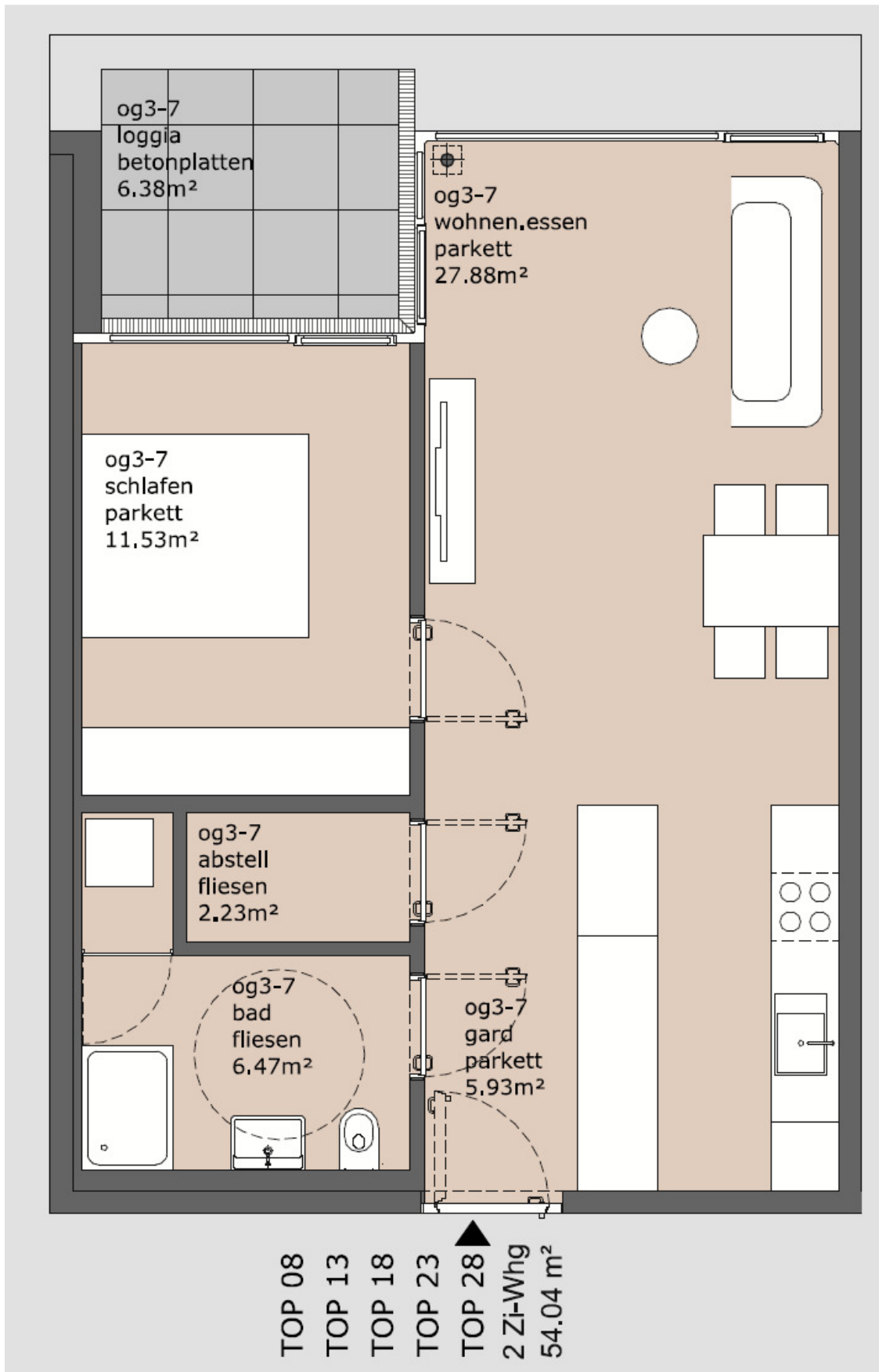
Grundriss der Tops 8, 13, 18, 23 und 28
