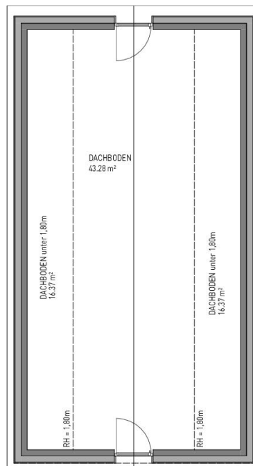
DACHGESCHOSS
