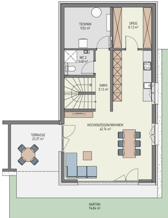
UNTERGESCHOSS
