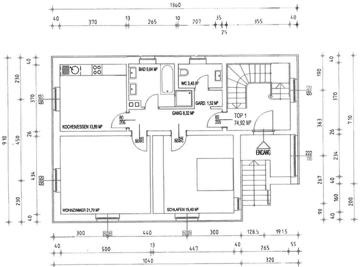
GRUNDRISS ERDGESCHOSS M1:100
