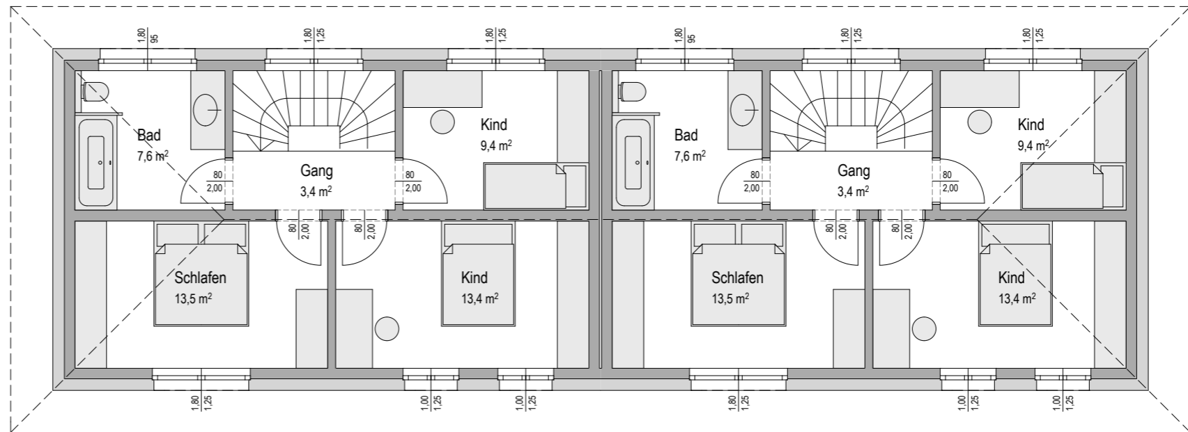
OBERGESCHOSS
