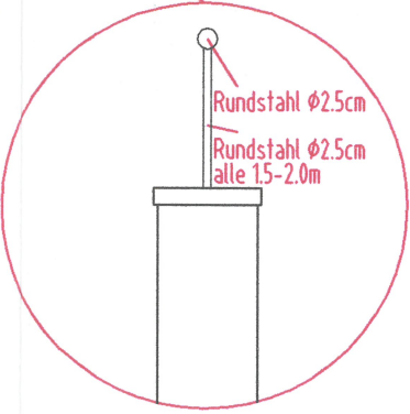
Detail Stiegenbrüstung und Handlauf M 1:10
