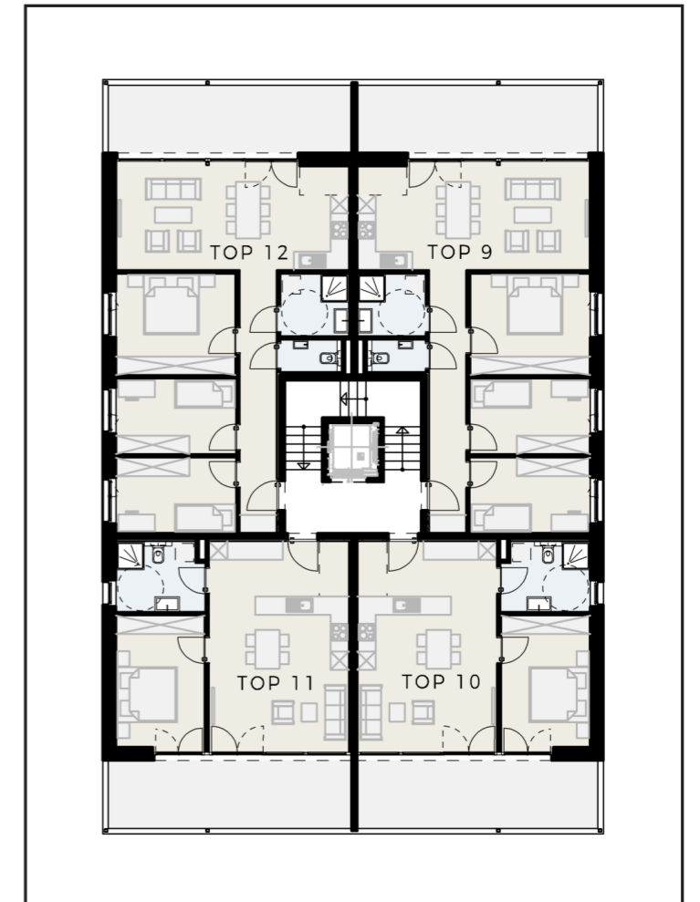
DACHGESCHOSS
