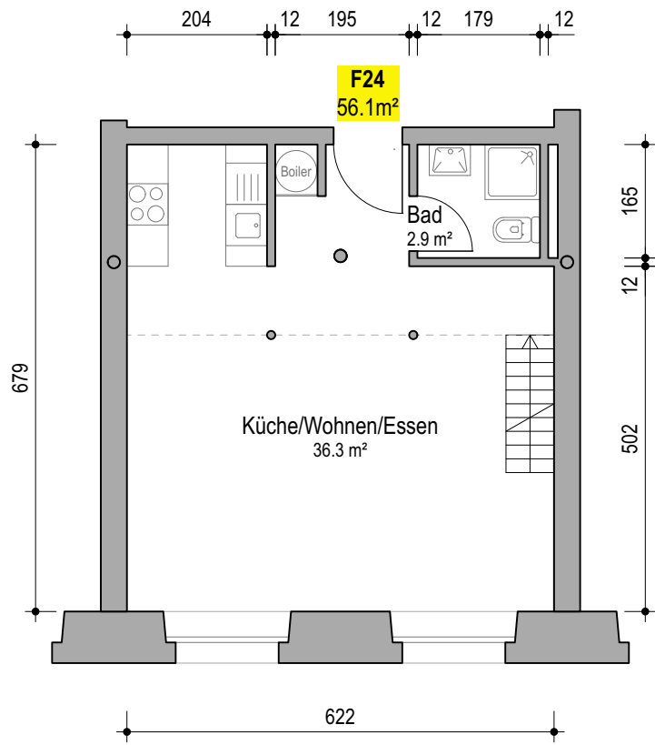
Top F24 Wohnung Mst. 1:100
