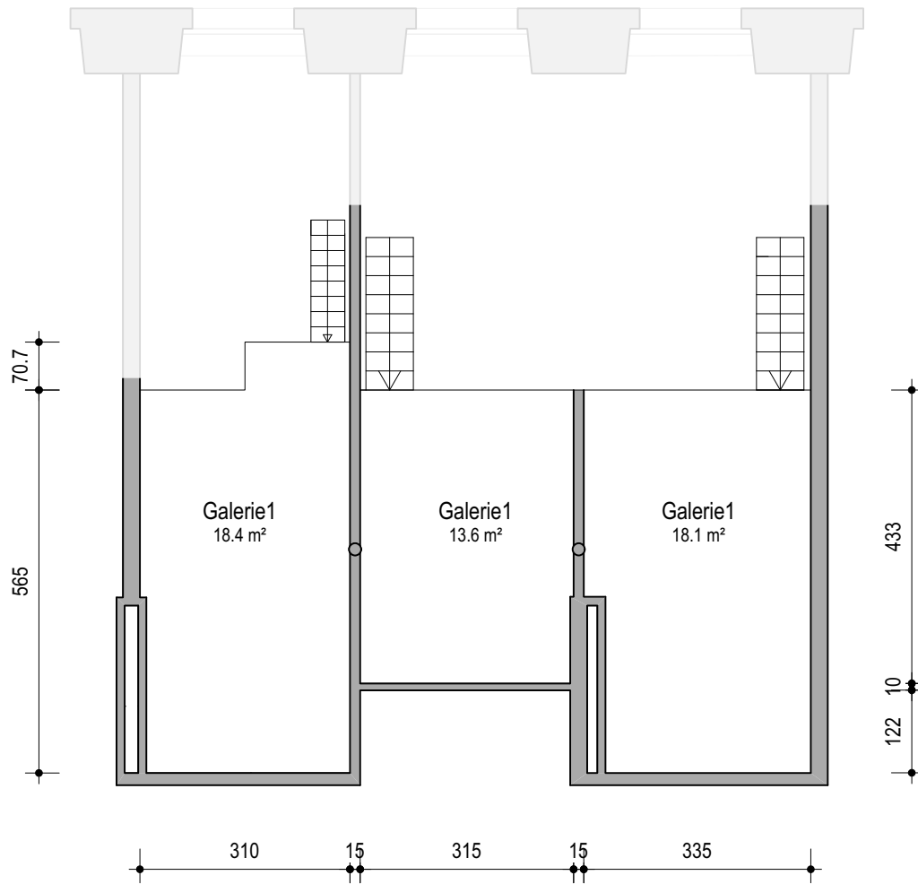
Top F10 Galerie Mst. 1:100
