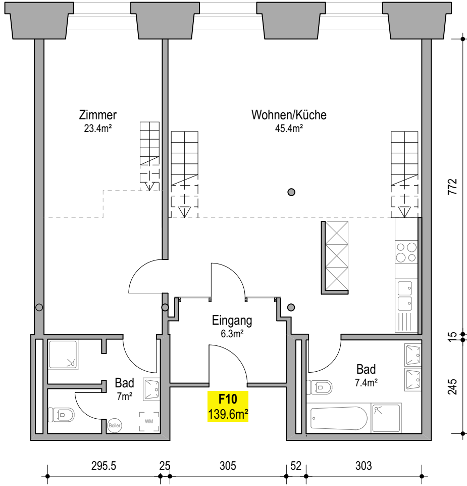
Top F10 Wohnung Mst. 1:100
