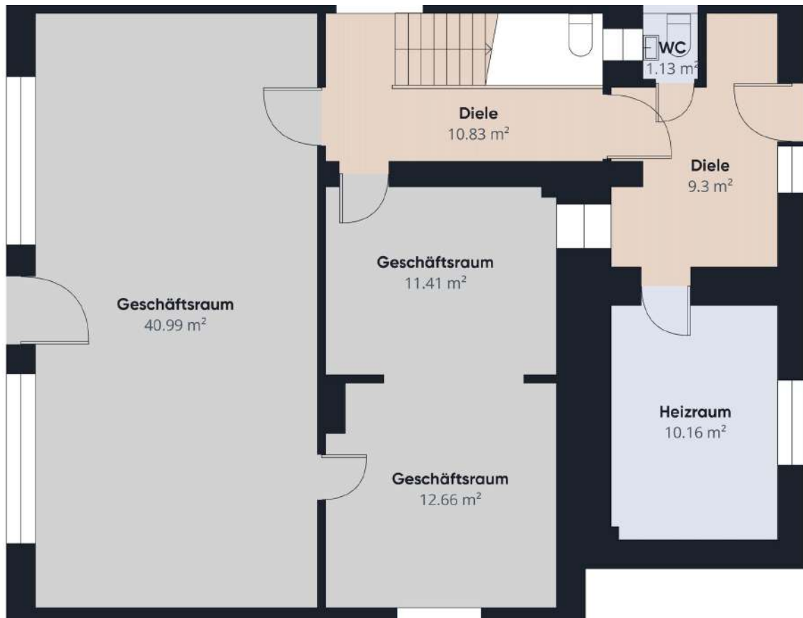
Grundriss EG ohne Maßstab
