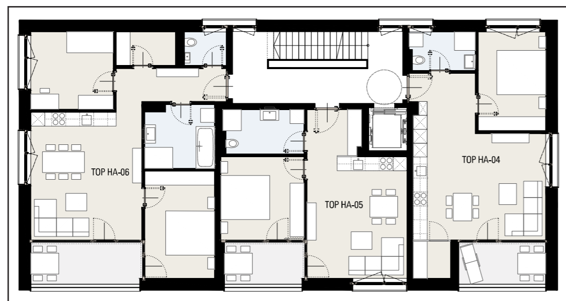
OBERGESCHOSS
