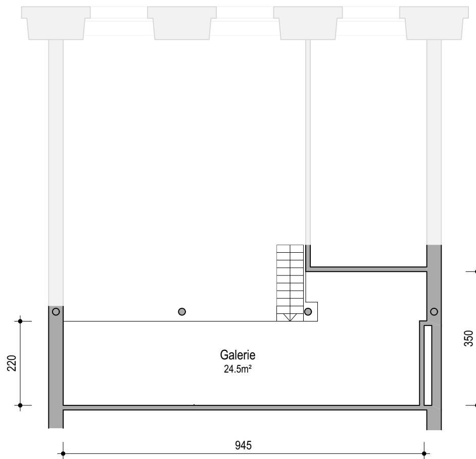
Top F23 Galerie Mst. 1:100
