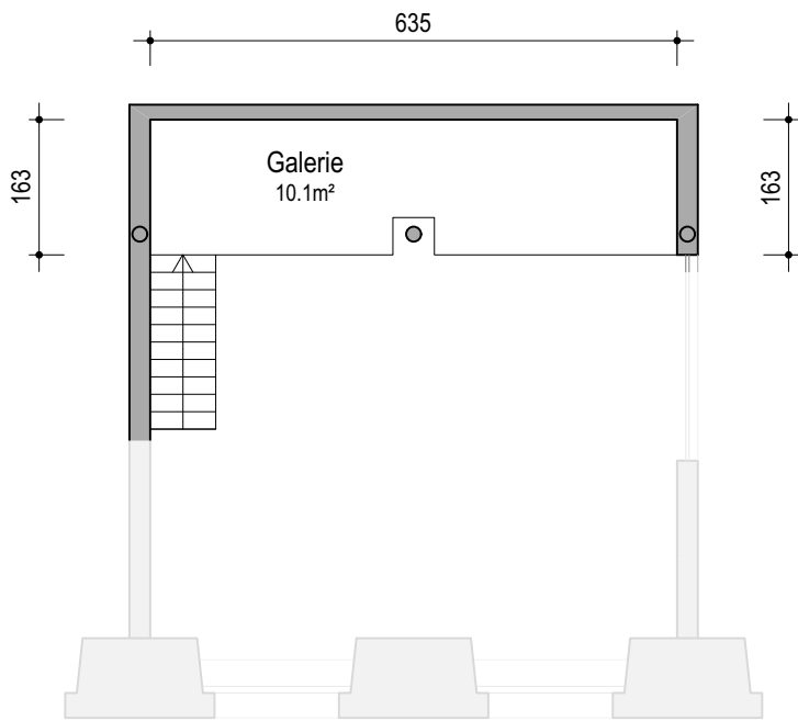
Top F11 Galerie Mst. 1:100
