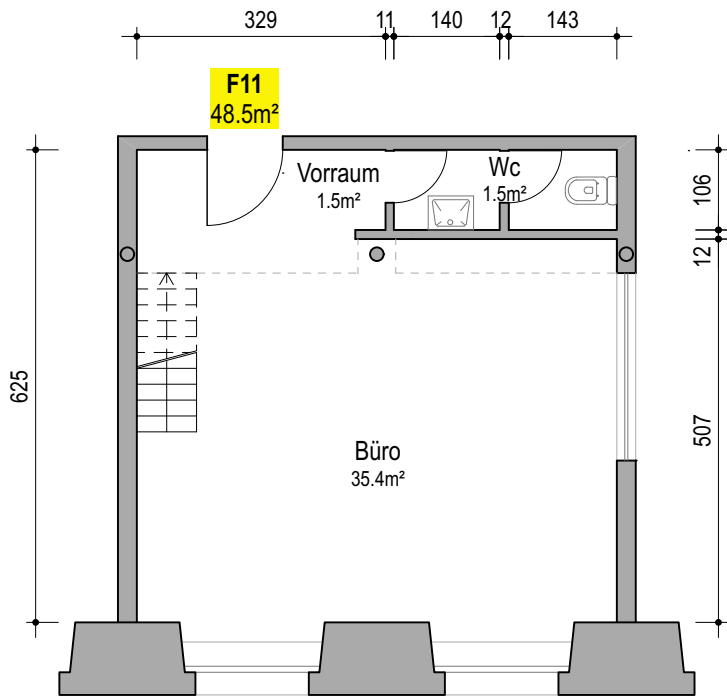
Top F11 Büro Mst. 1:100
