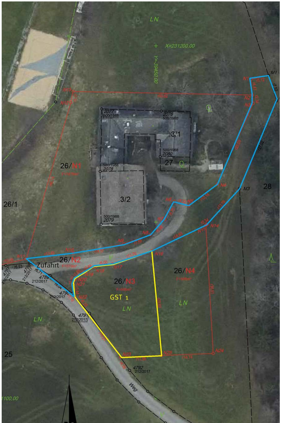
Teilungsplan Grundstück 1_Zufahrt_Maßstab 1:500
