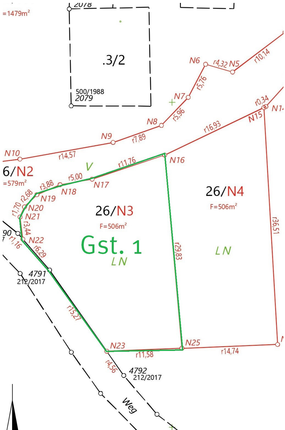
Teilungsplan Grundstück 1_Maßstab 1:500
