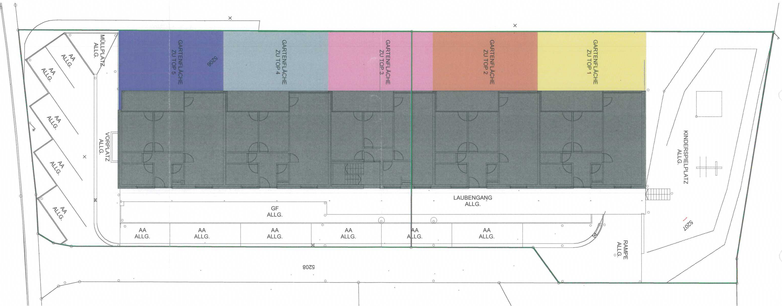
PLANBEILAGE ZUR NUTZWERTBERECHNUNG LAGEPLAN M 1:200
