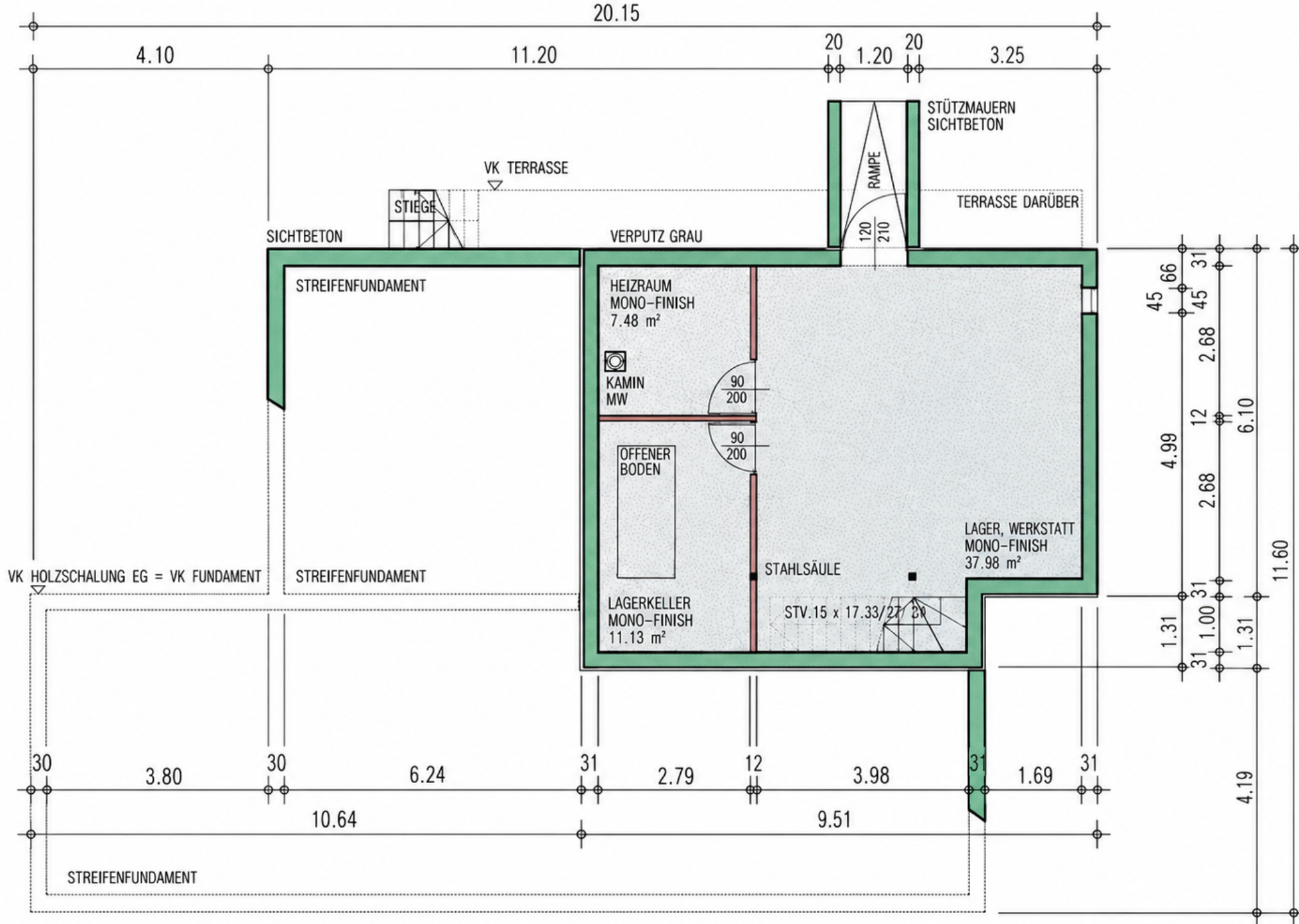
KELLERGESCHOSS M 1:100
