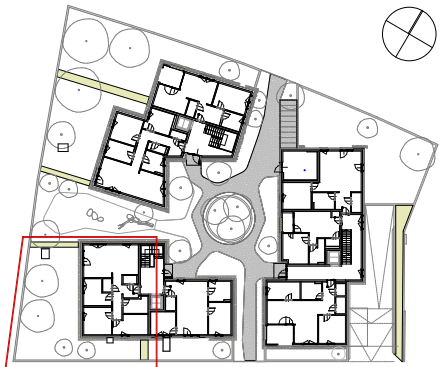
Übersicht Erdgeschoss
