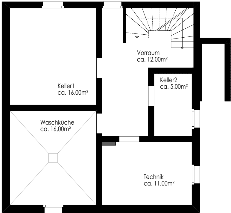
Untergeschoss M 1_100
