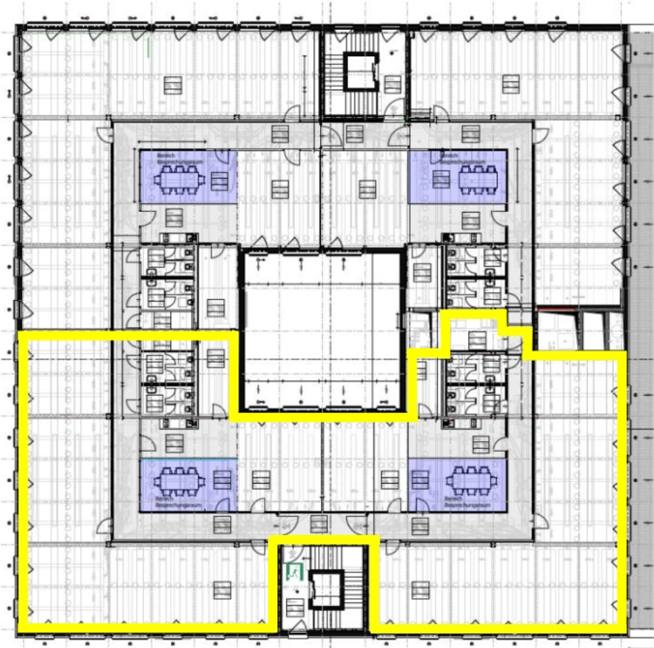
GRUNDRISS 3.OG - markierte Fläche mit ca. 591 m 2
