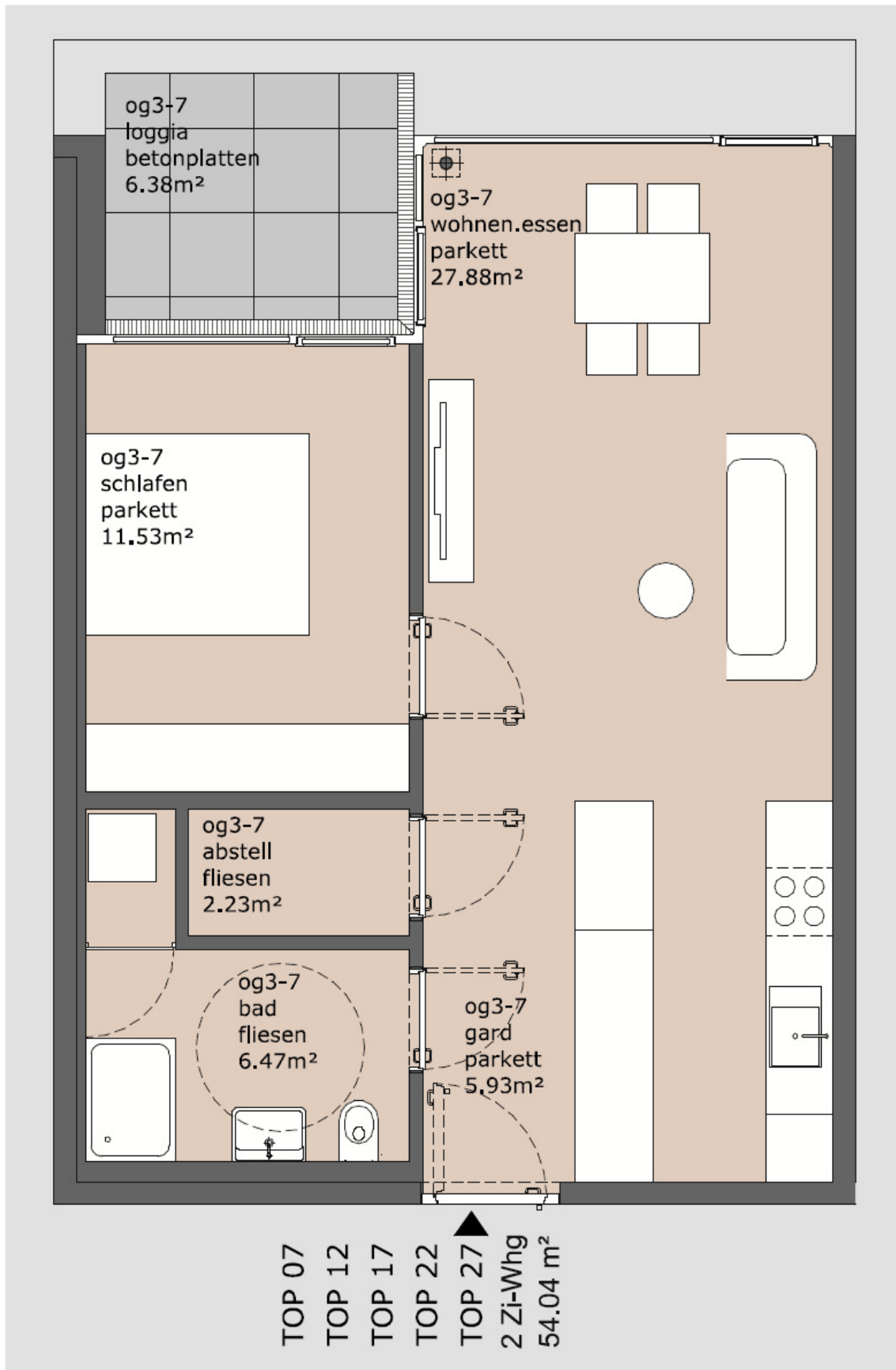
Grundriss der Tops 7, 12, 17, 22 und 27
