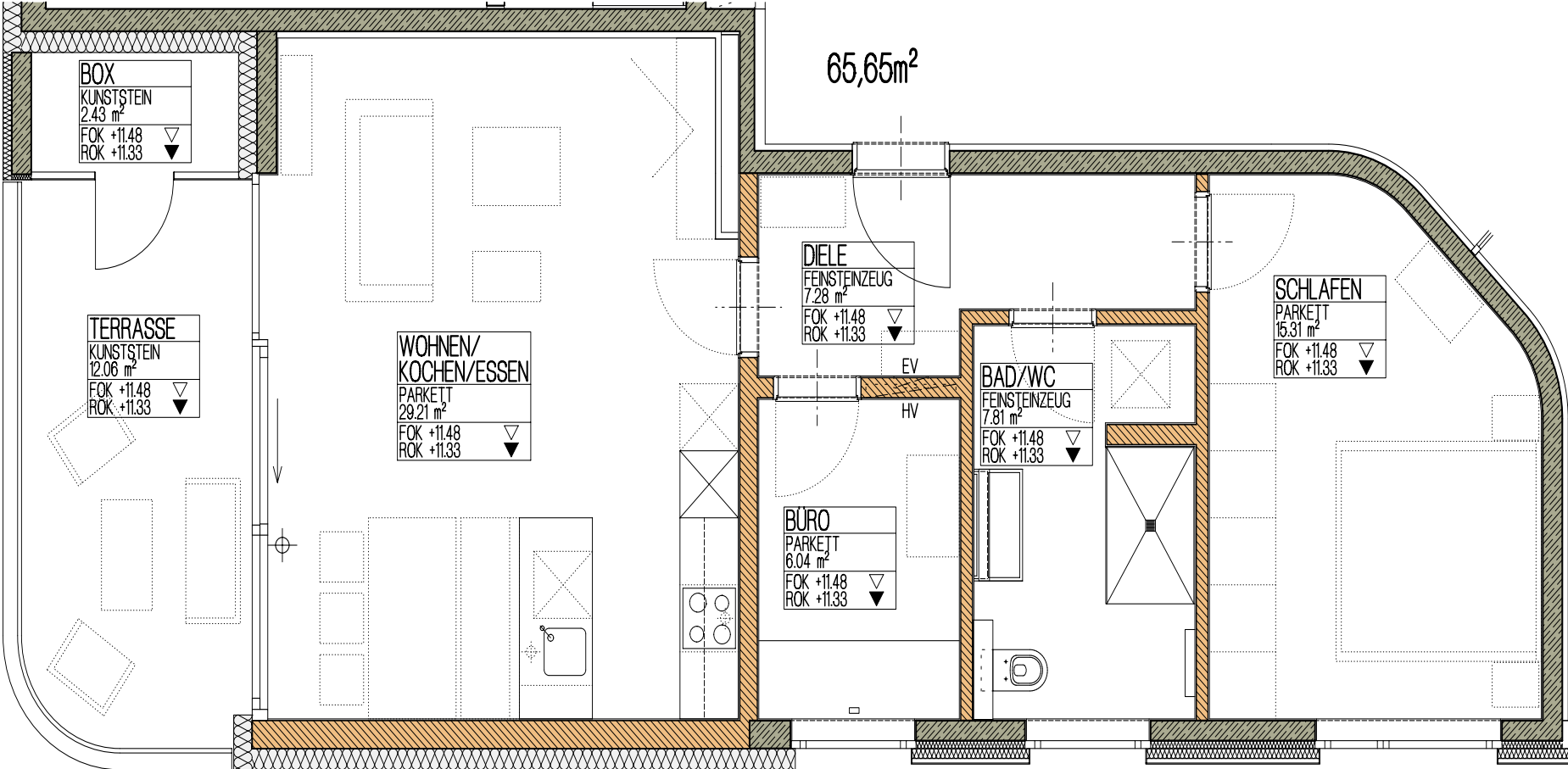
Grundriss Top 16 4. Obergeschoss
