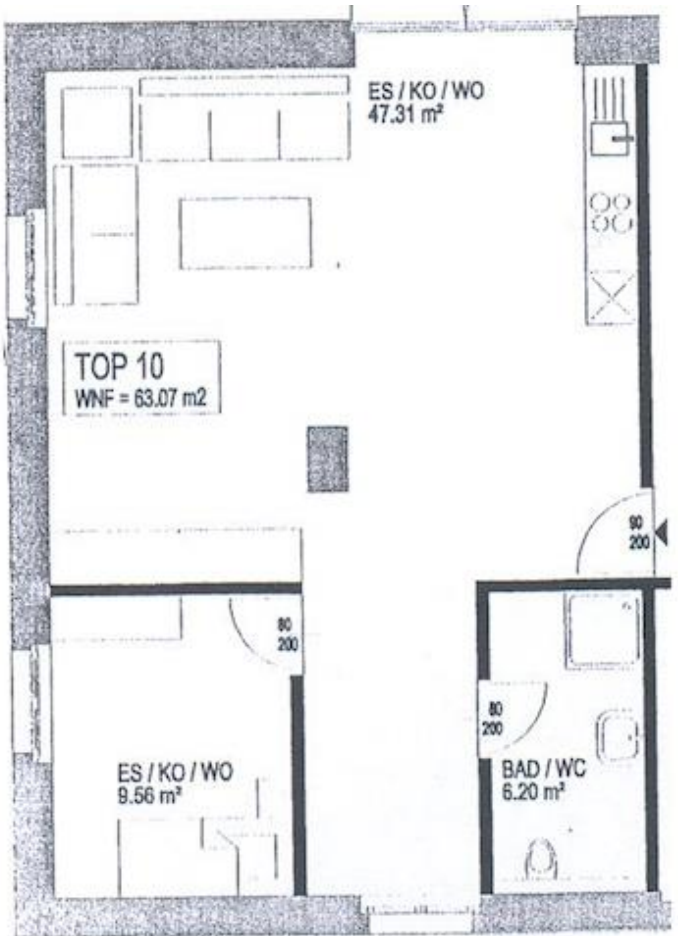
Grundriss
