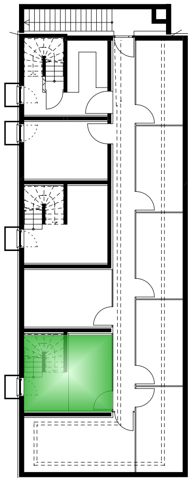
Kellergeschoss M 1/200
