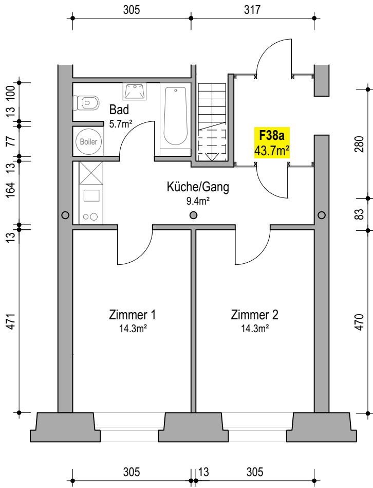
Top F38a Wohnung Mst. 1:100
