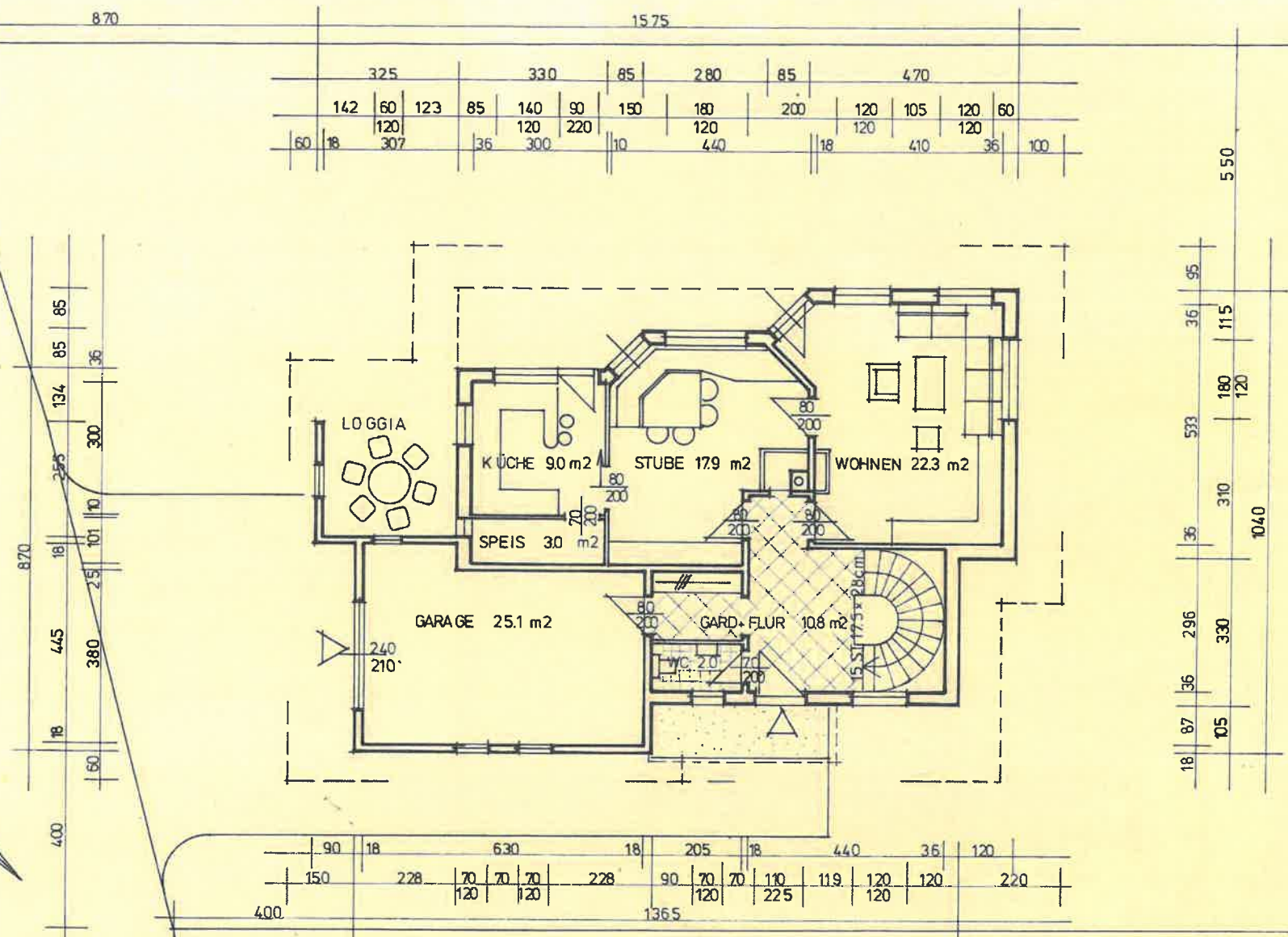
ERDGESCHOSS 1 : 1000
