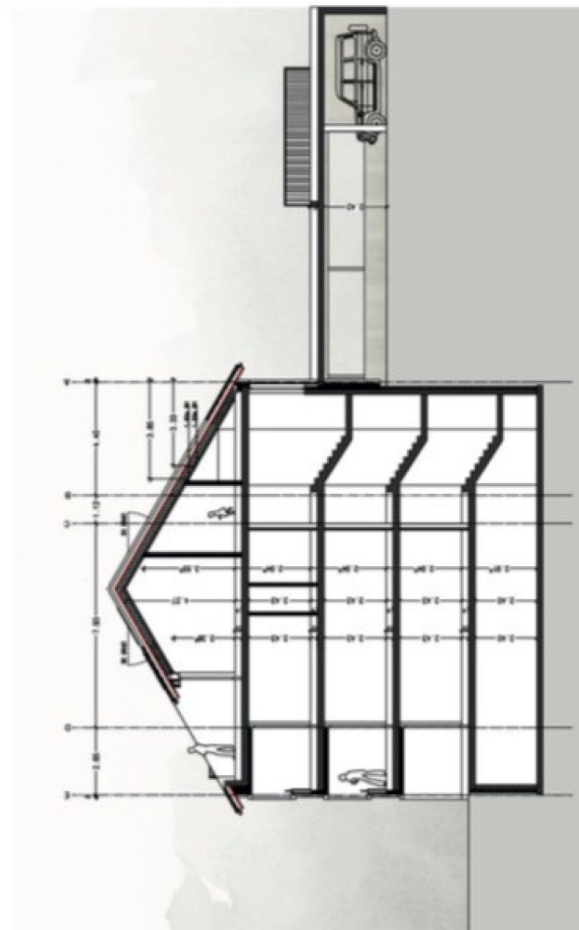
SCHNITT 1-1
