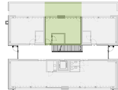
Übersicht EG
