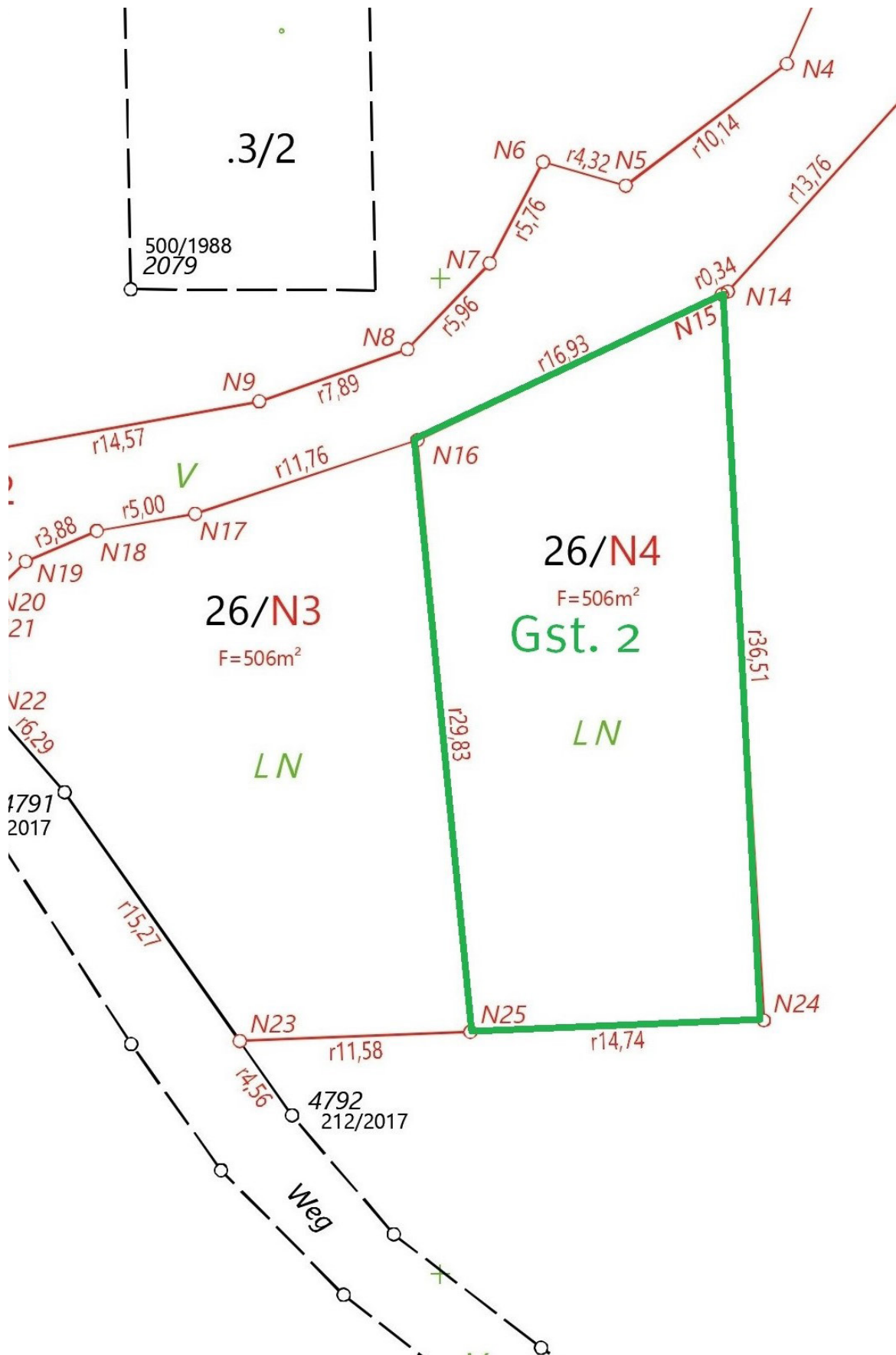
Teilungsplan Grundstück 2_Maßstab 1:500
