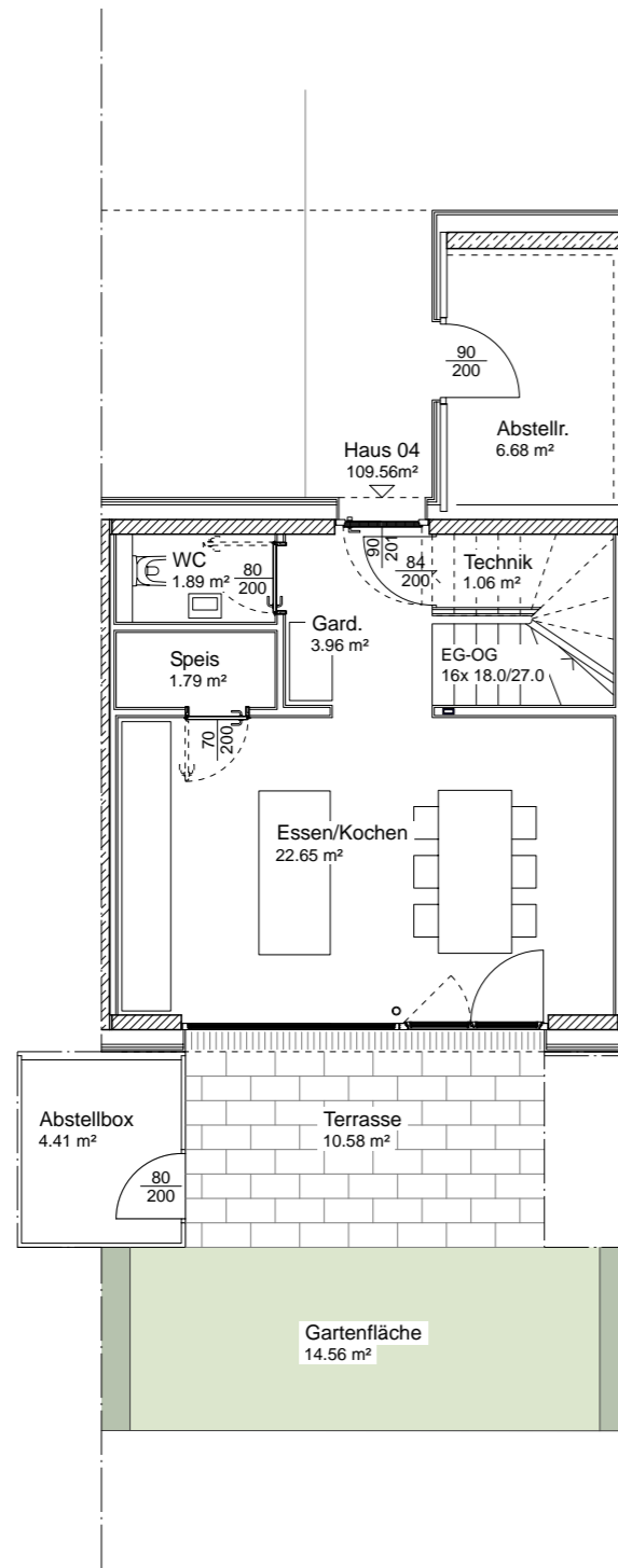
Grundriss Erdgeschoss
