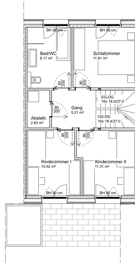
Grundriss Obergeschoss
